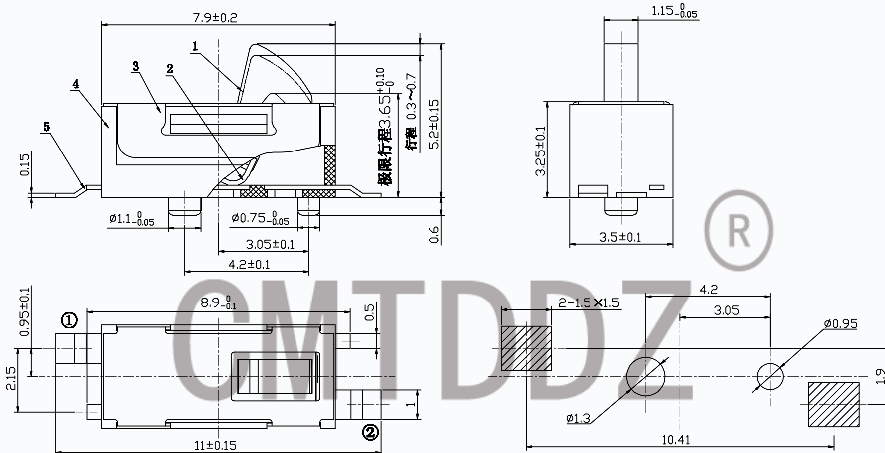
安装尺寸图
