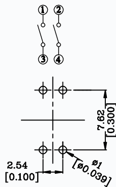
P.C.B LAYOUT
